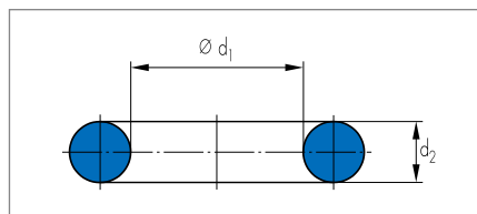
符合DIN 3771-第一部分的设计, 质量为“N”
