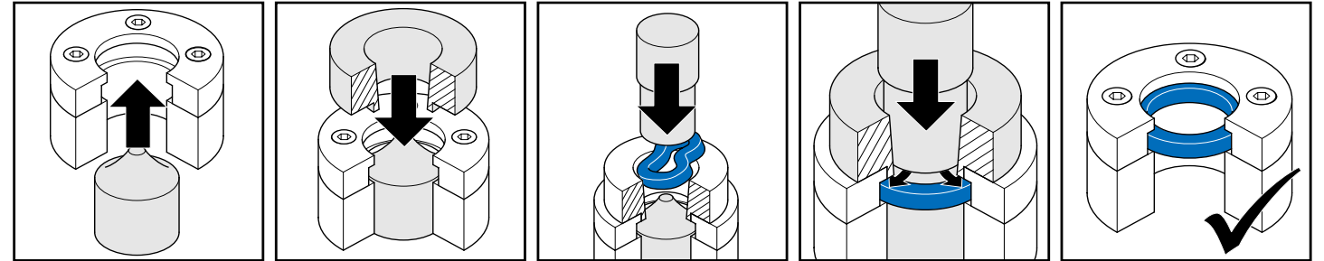
1B. 通过压装工具、定位锥套和辅助压板进行安装
