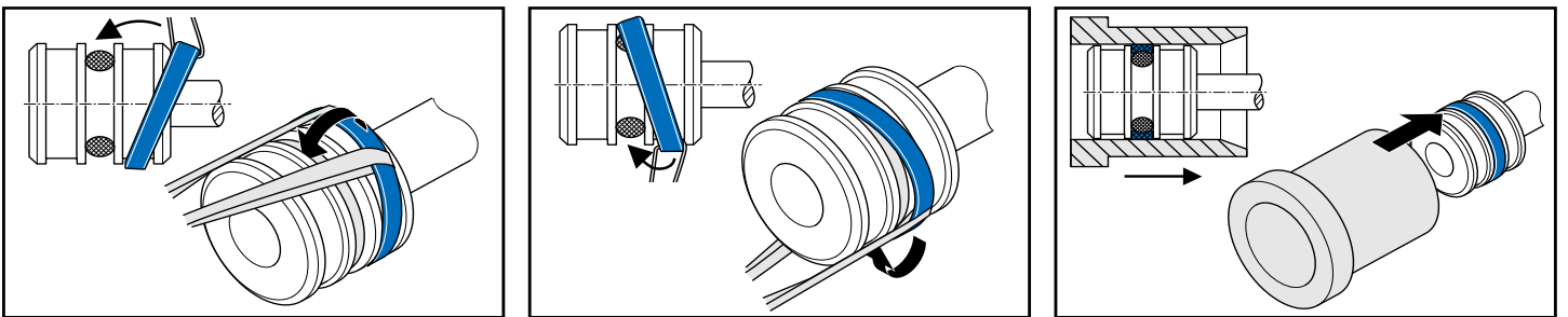
2. 通过安装带及校准套筒进行安装
