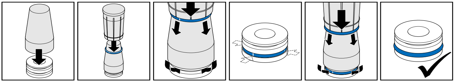
1. 通过膨胀锥套与定位锥套进行安装
